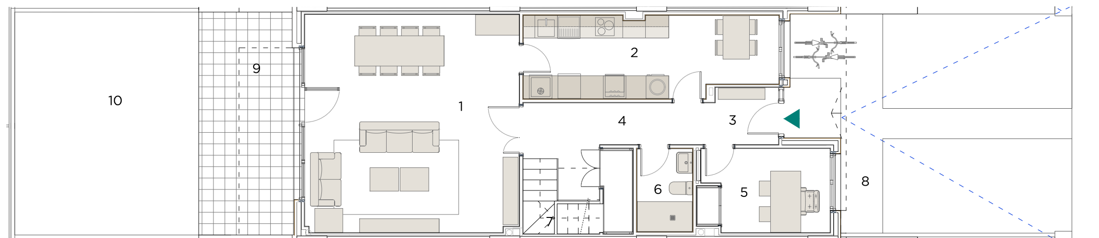
PLANTA BAJA
